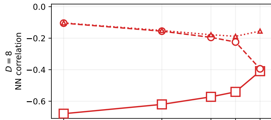
Dimer-plaquette pin
