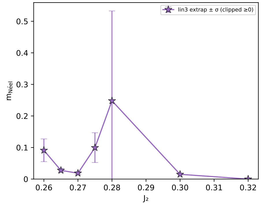
C6Y \pi
