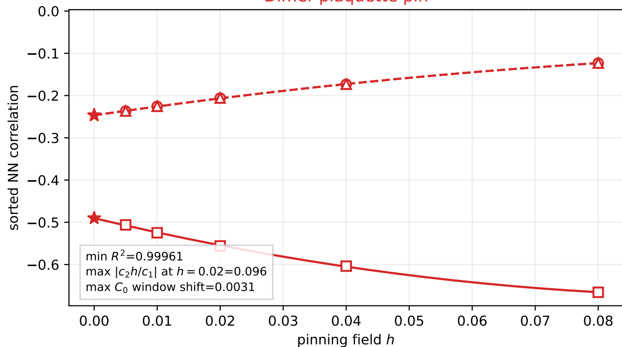
Dimer-plaquette pin
