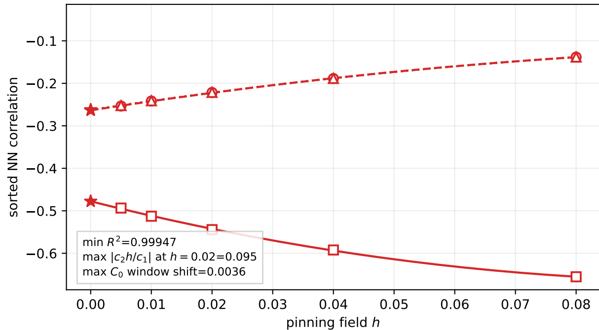
Dimer-plaquette pin
