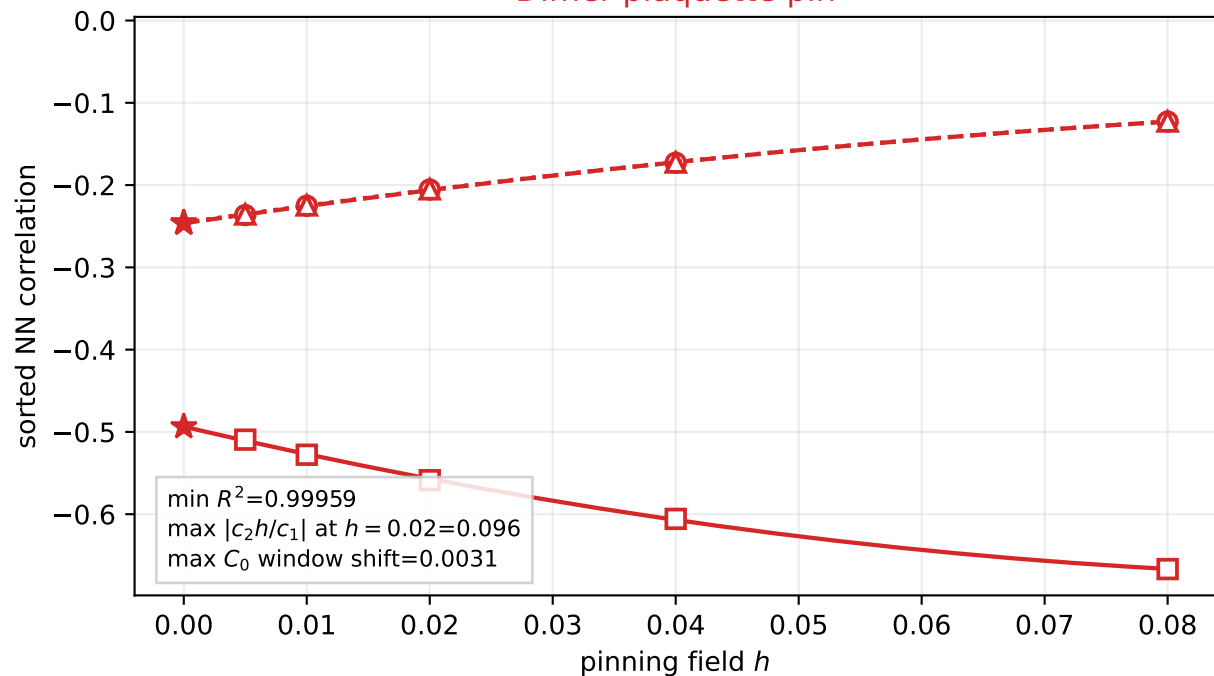
Dimer-plaquette pin
