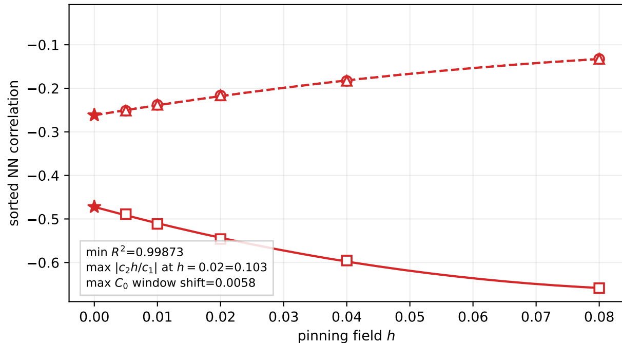
Dimer-plaquette pin
