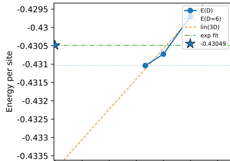
Néel
