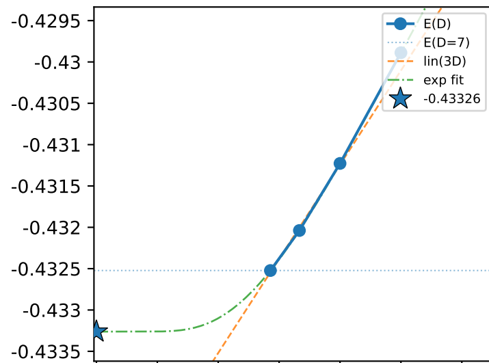
C6Y \pi
