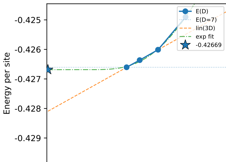
Néel
