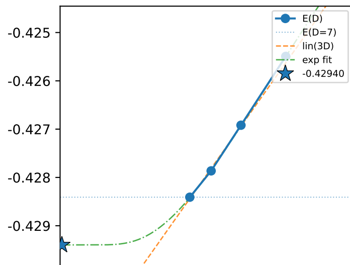
C6Y \pi
