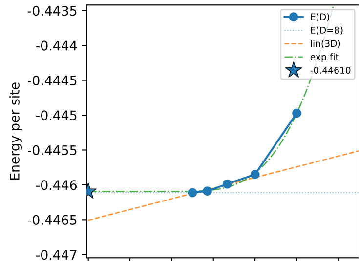
Néel
