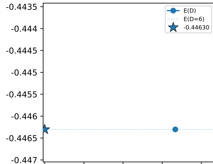
2 C3
