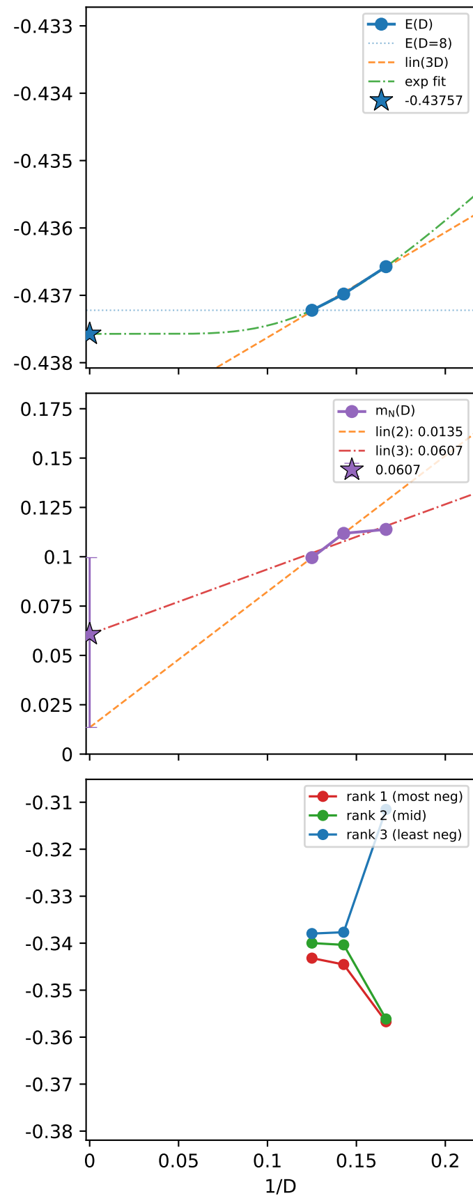
2 C3
