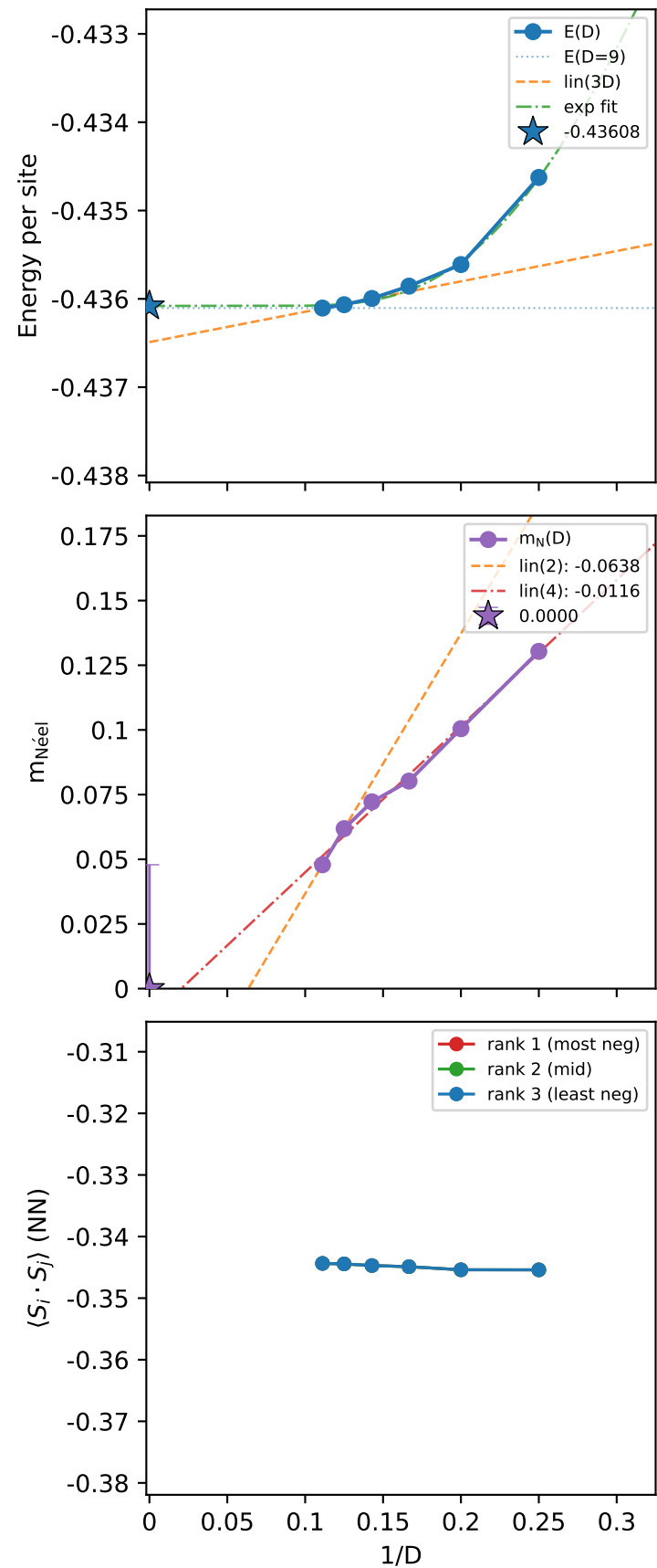
Néel
