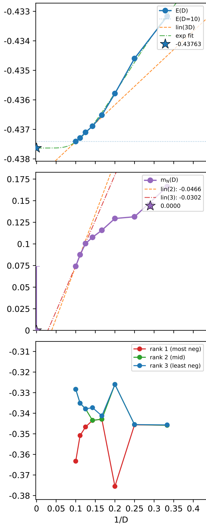
C6Y \pi
