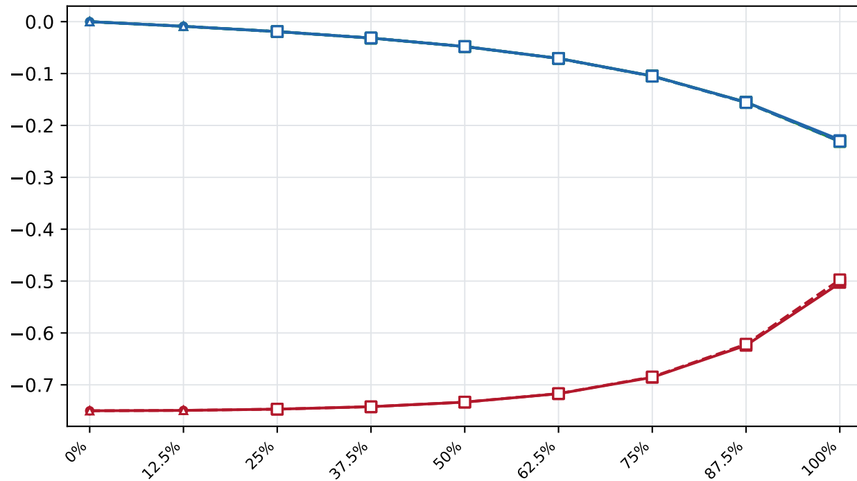
Dimer
