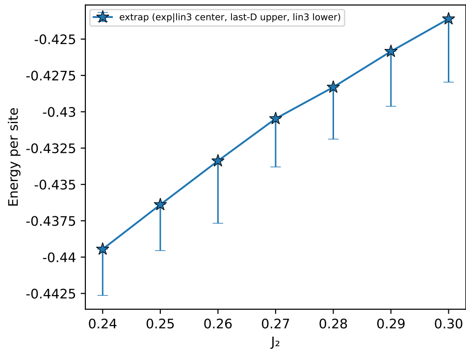
2 C3
