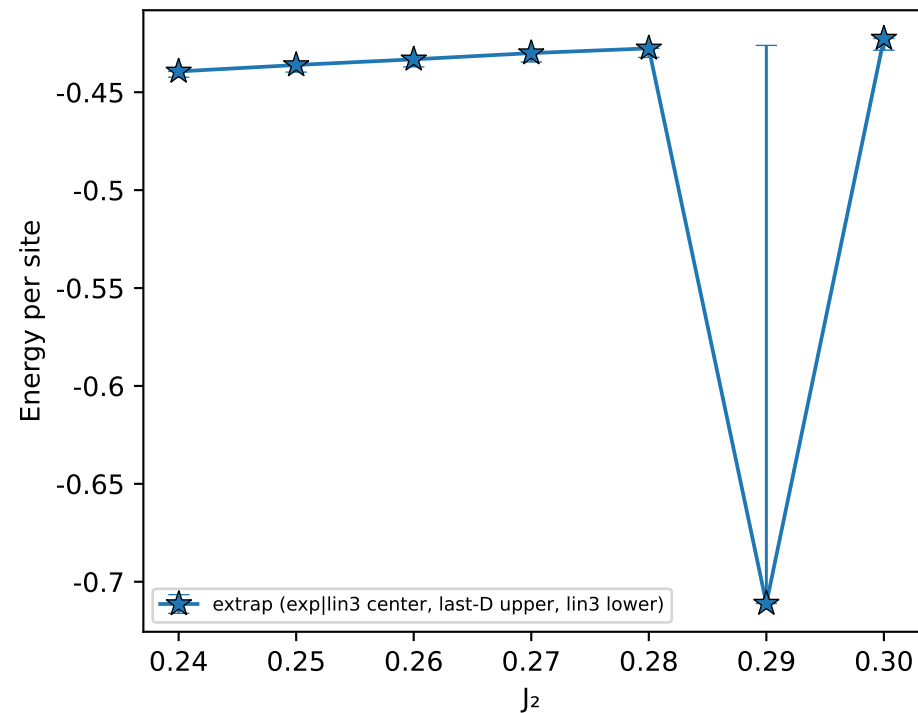
C6Y \pi
