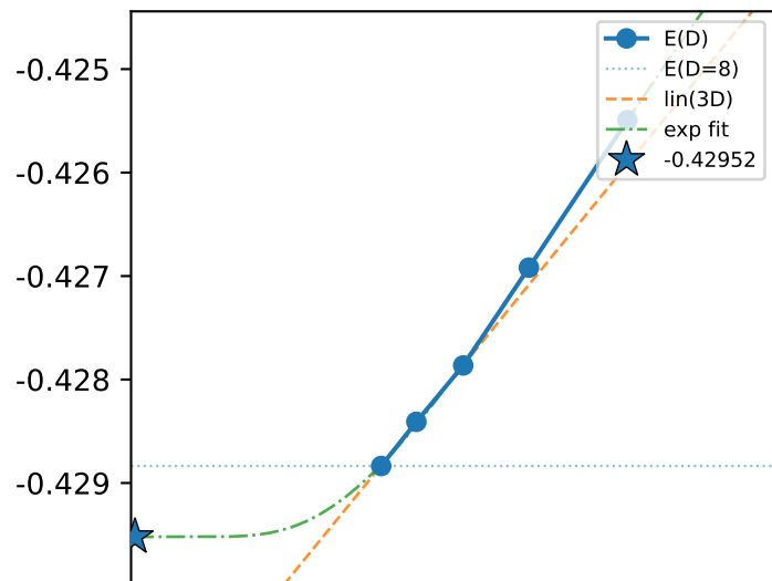
C6Y \pi
