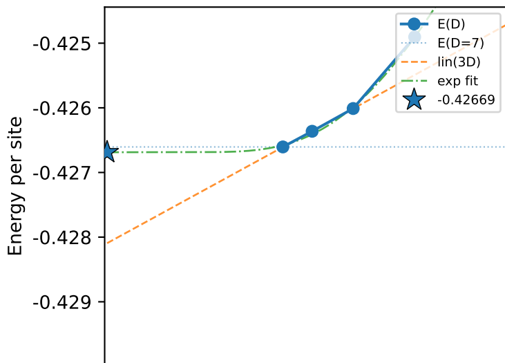
Néel
