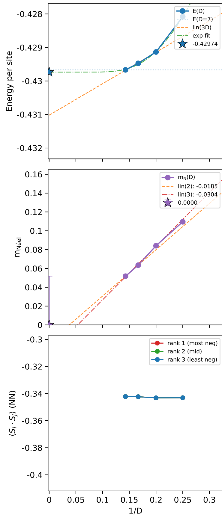
Néel
