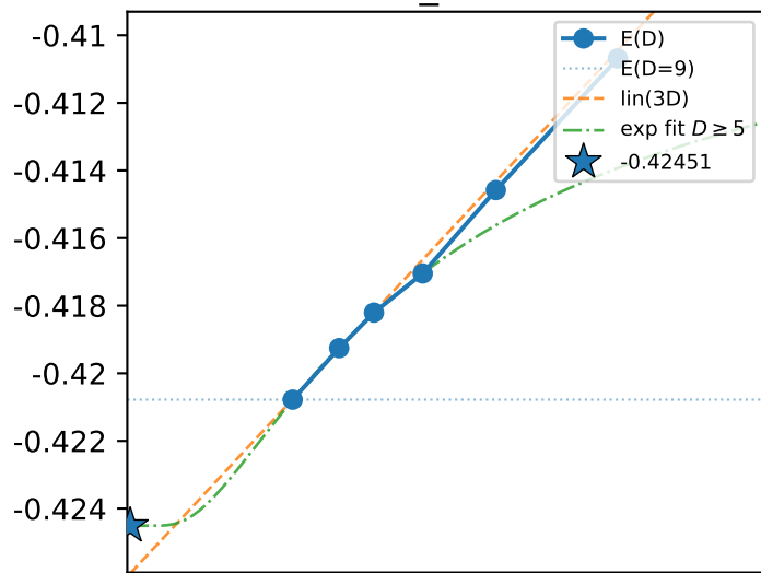
2tensor_columnar
