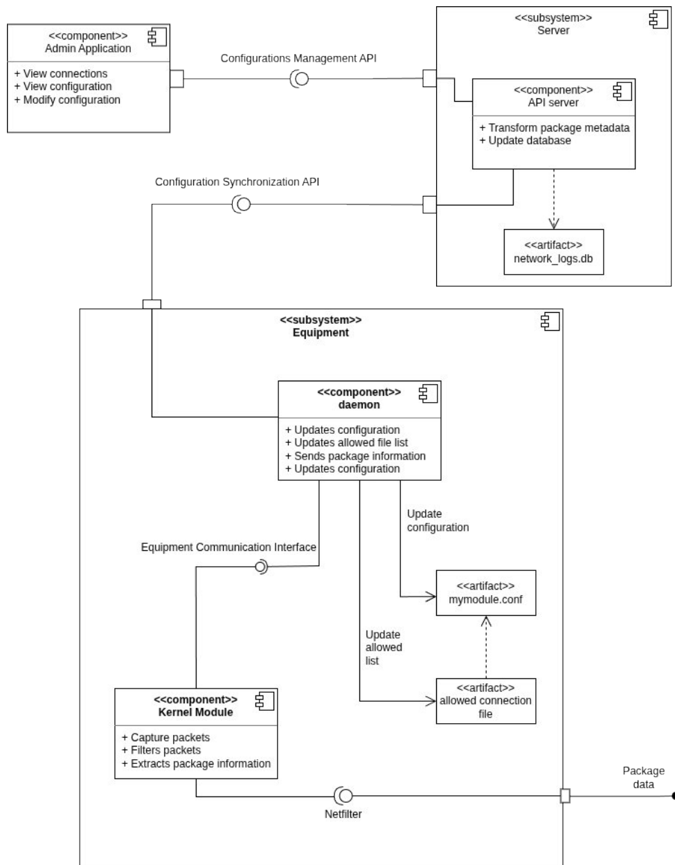
Imagine 1 Diagramă de componente
