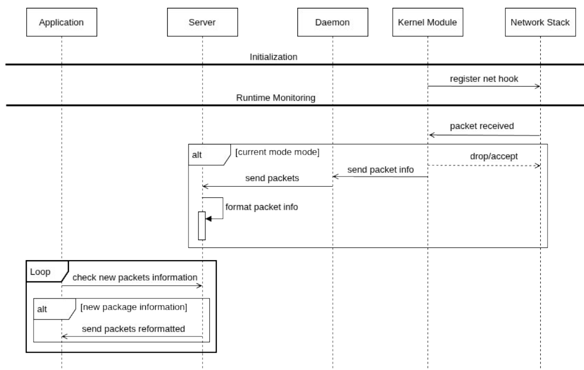
Imagine 3 Diagramă secvențială - configurații
