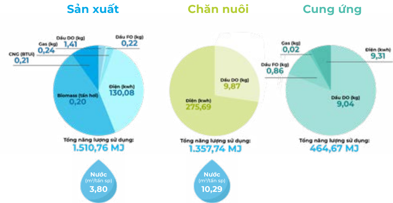
CƠ CẤU SỬ DỤNG NĂNG LƯỢNG - TÀI NGUYÊN TRÊN TẤN SẢN PHẨM TRONG CHUỖI HOẠT ĐỘNG SẢN XUẤT - CHĂN NUÔI - CUNG ỨNG 2018
