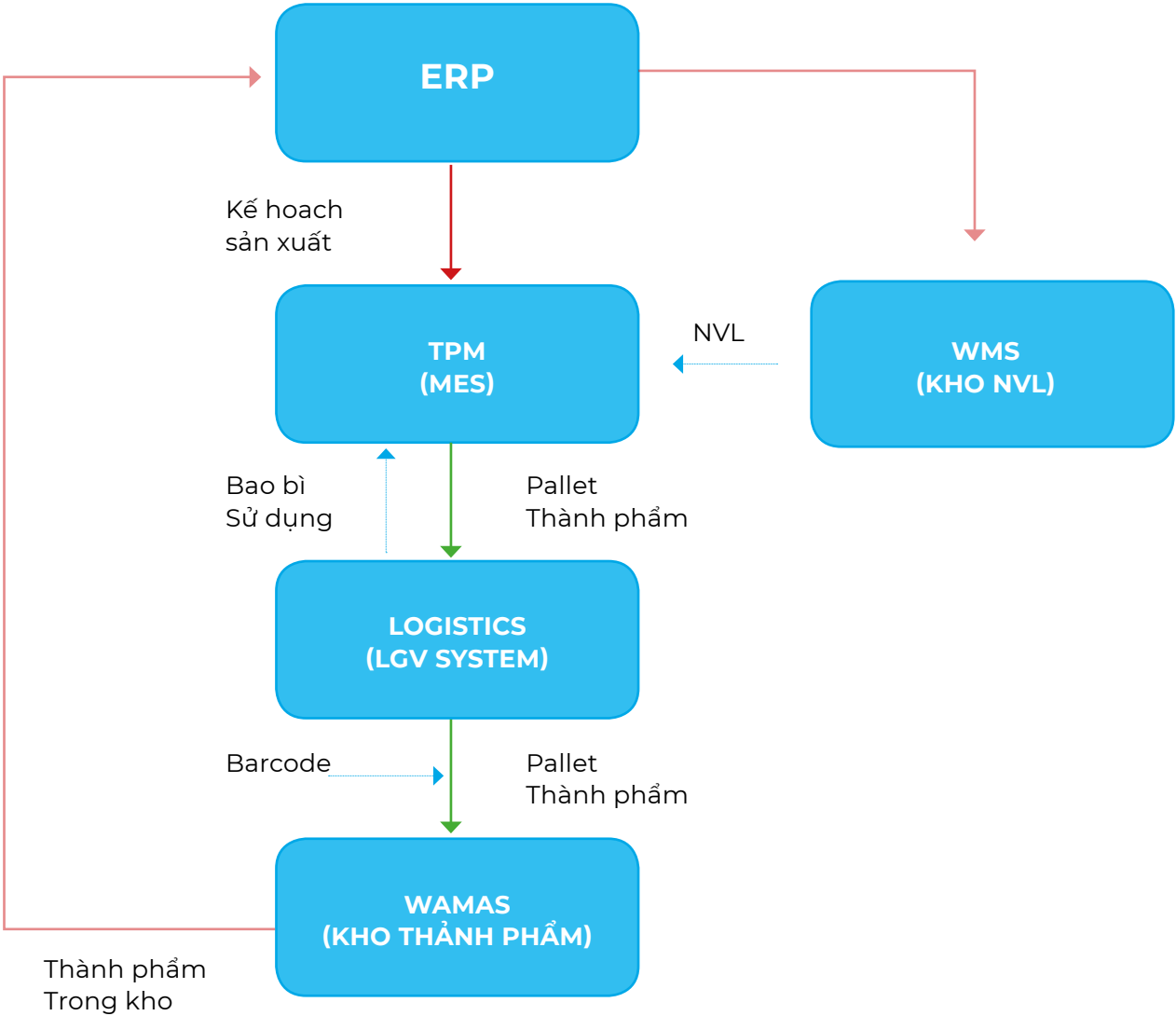
Mô phỏng hoạt động hệ thống MES tại Nhà máy Sữa Việt Nam
