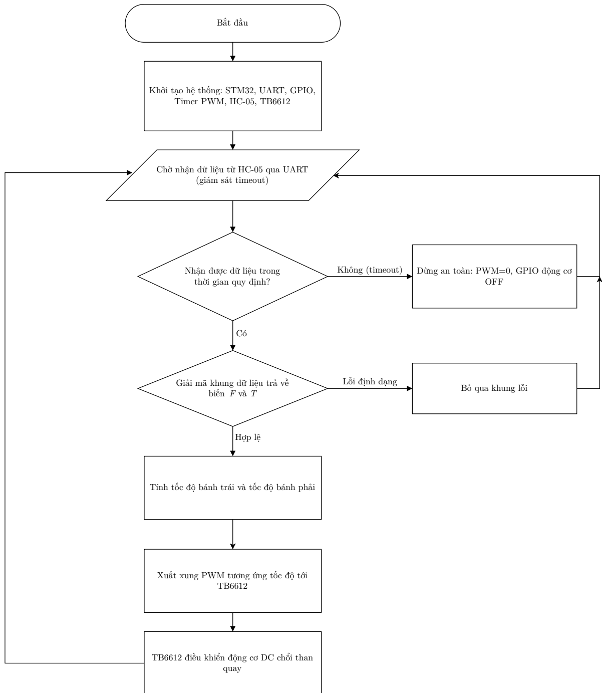
Hình 2.5: Lưu đồ giải thuật chi tiết của khối thu
