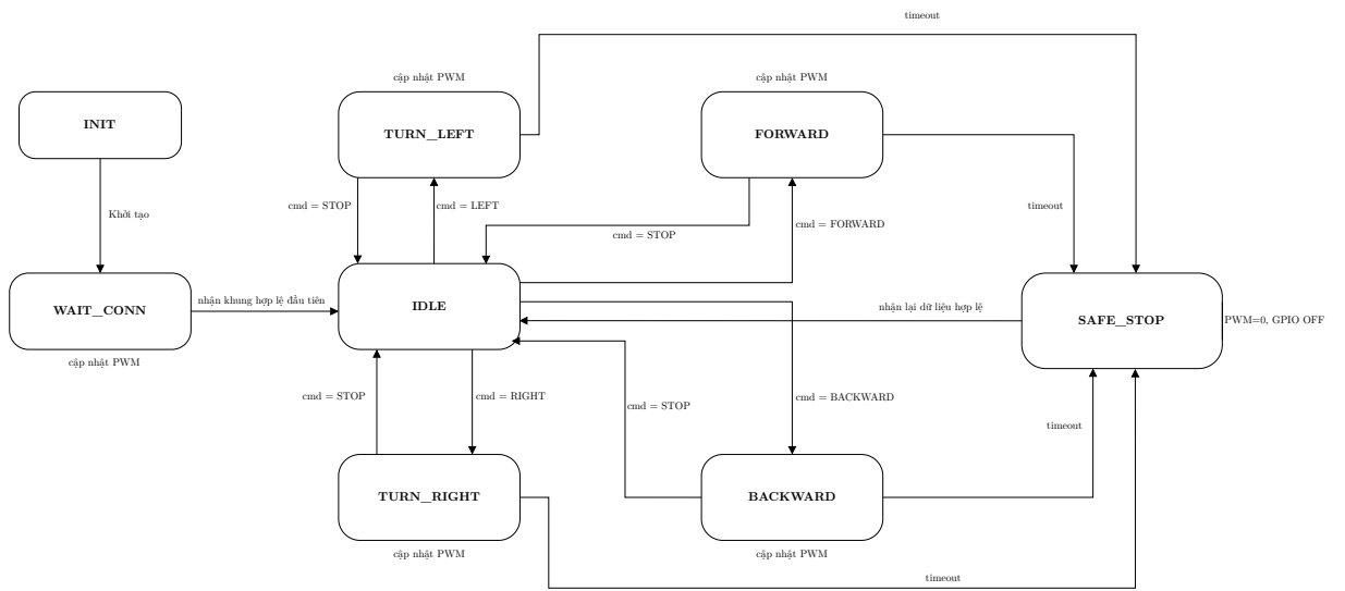
Hình 2.7: Sơ đồ máy trạng thái khởi thu
