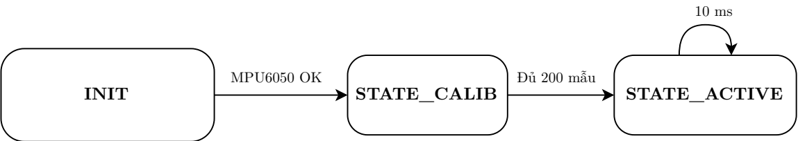
Hình 2.6: Sơ đồ máy trạng thái khối phát
