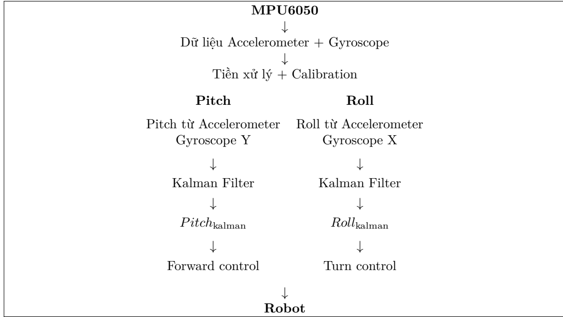
Hình 3.5: Luồng xử lý dữ liệu từ MPU6050 đến điều khiển robot
