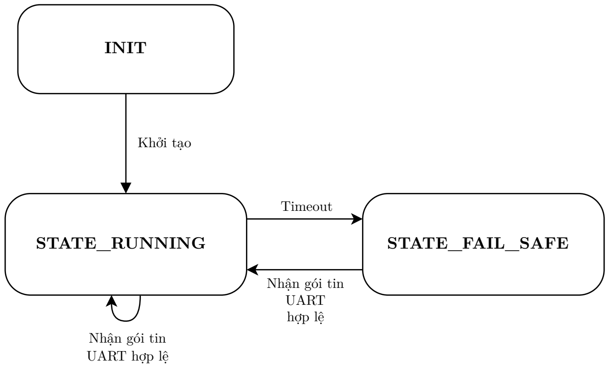
Hình 2.7: Sơ đồ máy trạng thái khởi thu
