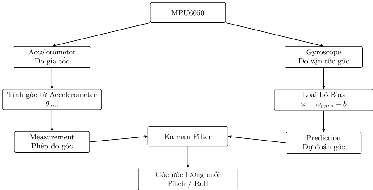
Hình 3.4: Luồng xử lý dữ liệu MPU6050 và triển khai Kalman Filter
