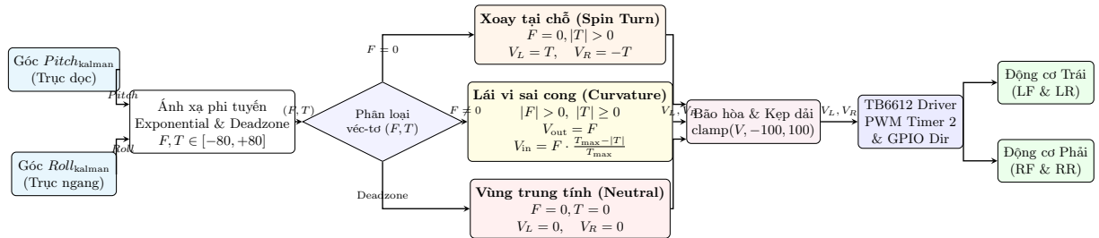
Hình 3.6: Sơ đồ khối cấu trúc giải thuật điều khiển lái vi sai cong thích nghi
