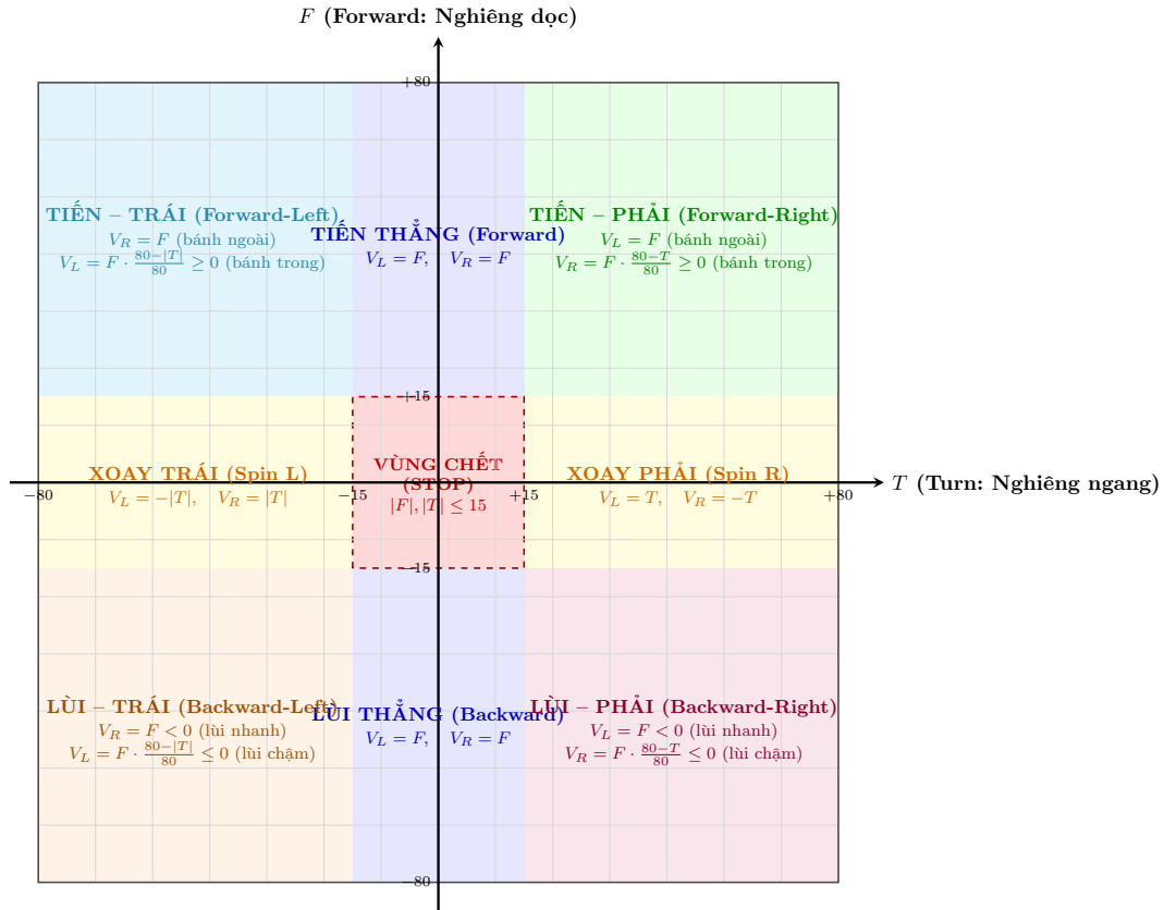
Hình 3.7: Không gian trạng thái điều khiển 8 hướng và phân bố vận tốc vi sai trong mặt phẳng pha (T, F)
