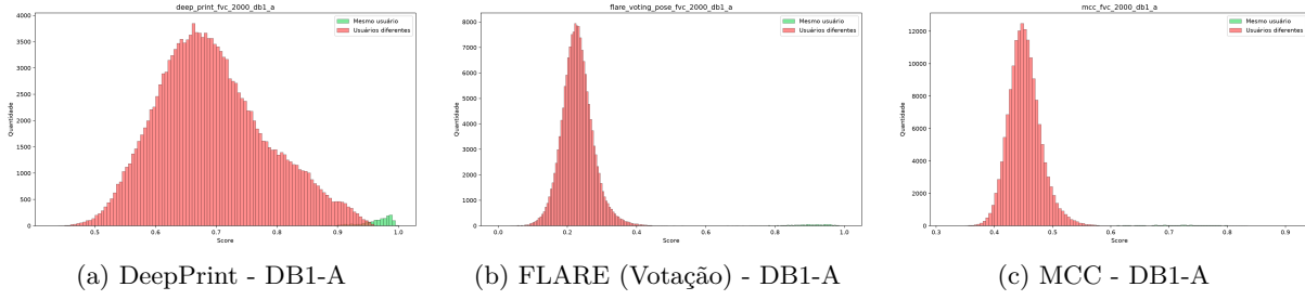
Figura 1 – Comparação da distribuição das pontuações de similaridade entre DeepPrint, FLARE com alinhamento por votação e MCC para o subconjunto DB1-A do FVC2000.
