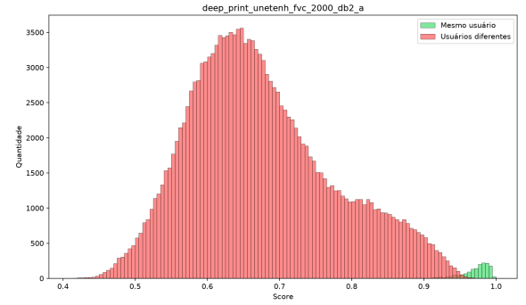
(d) DeepPrint + UNetEnh - DB2-A
