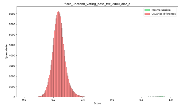
(h) FLARE (Votação) + UNetEnh - DB2-A
