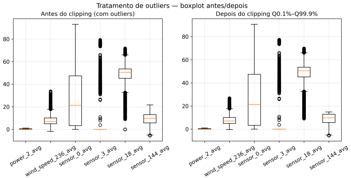
Figura 9: Boxplots antes e depois do clipping Q0,1%–Q99,9% por feature.
