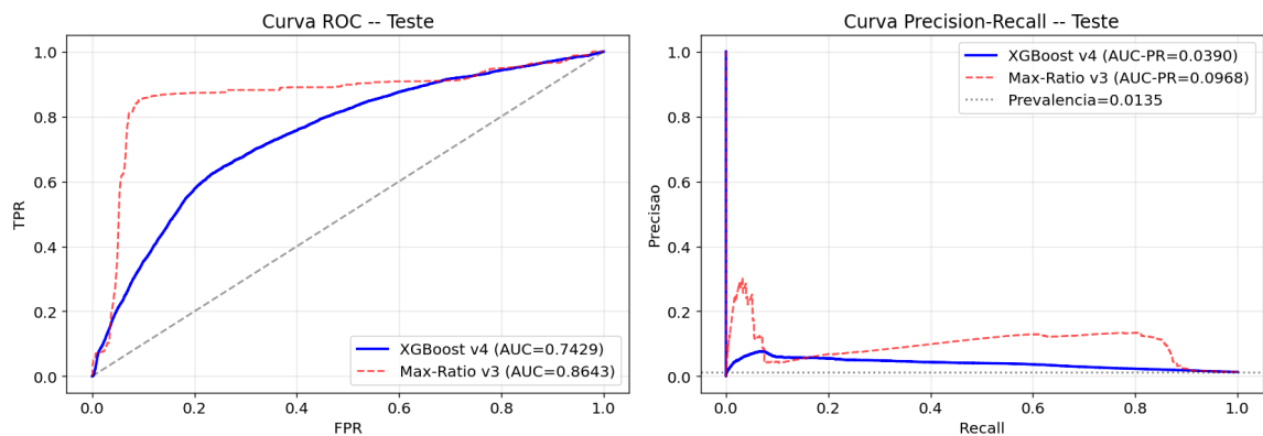
Figura 20: Curvas ROC e Precision-Recall do NB2.
