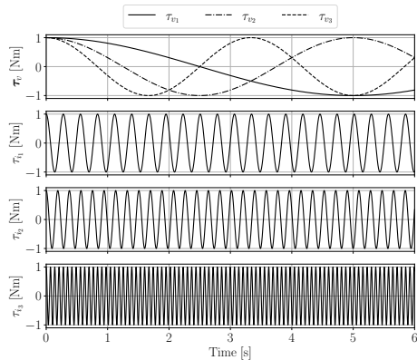
Torques voluntários (movimento) e de tremor.
