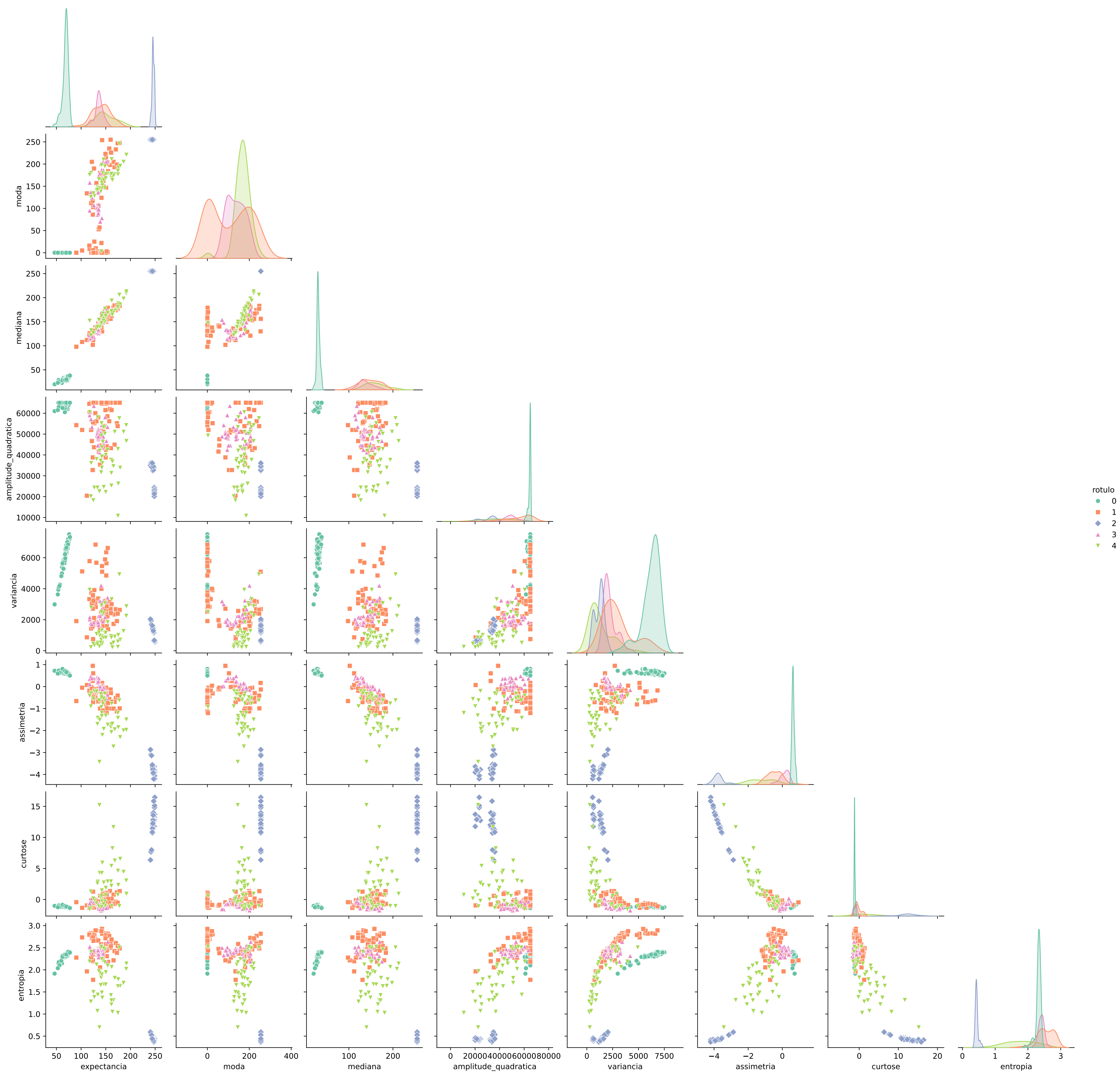
Dispersão das Features - trabalho_4_features_bins_8.csv
