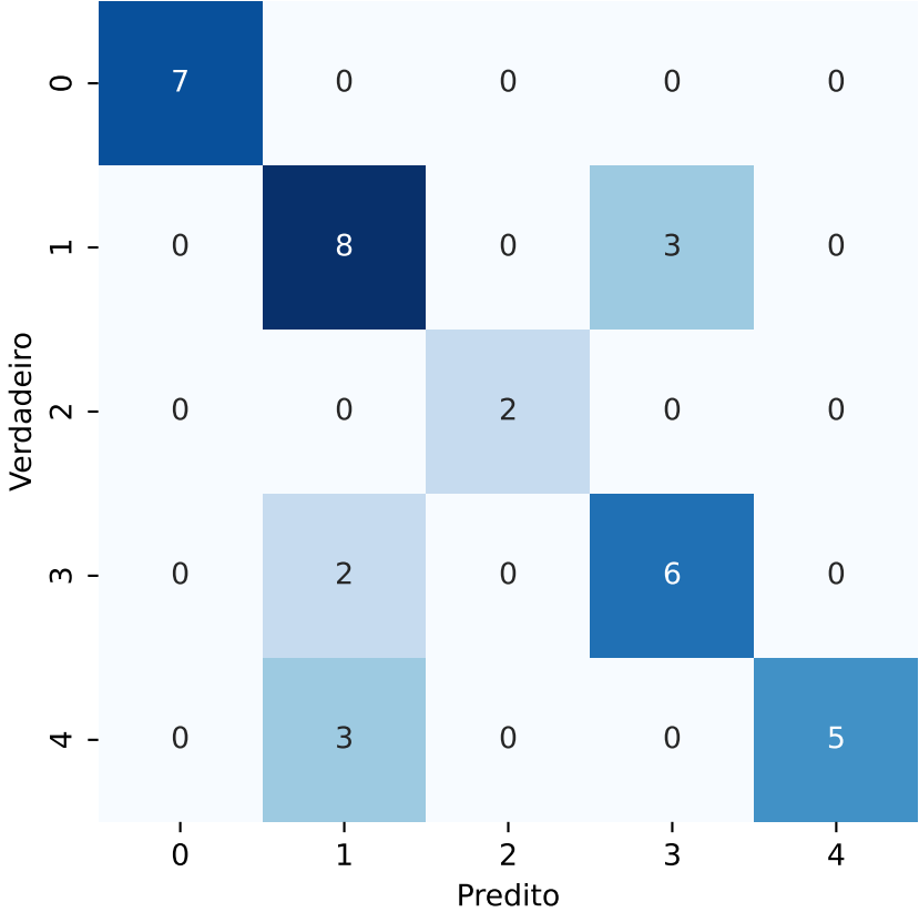
Matriz de Confusão - LDA - trabalho_4_features_bins_16-PARCIAL.csv
