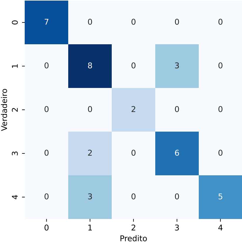
Matriz de Confusão - LDA - trabalho_4_features_bins_8-PARCIAL.csv
