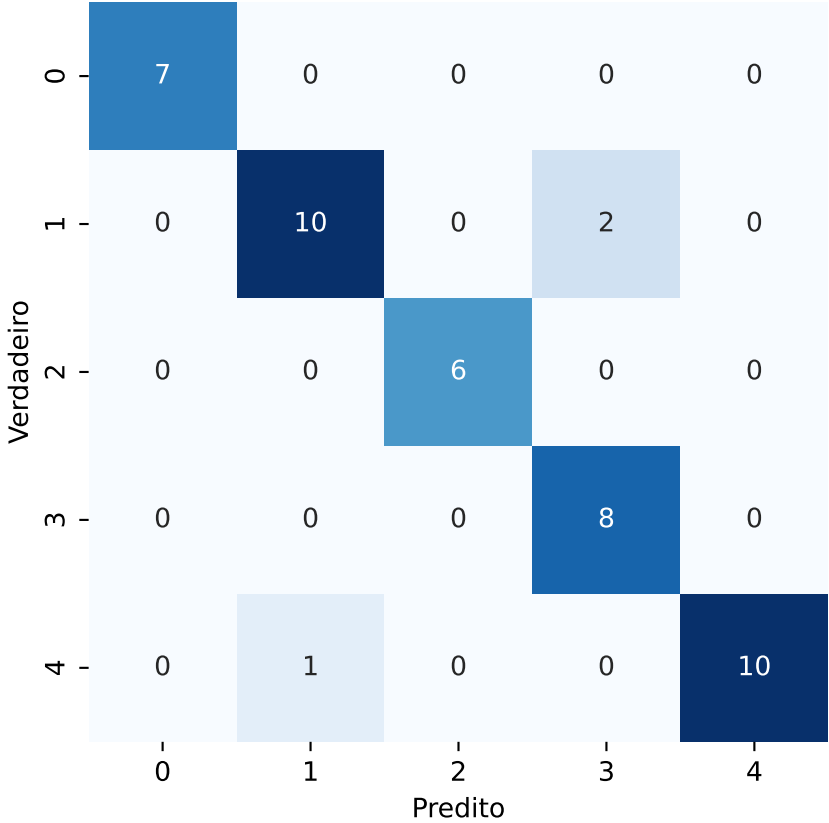
Matriz de Confusão - LDA - trabalho_6_features_bins_16-PARCIAL.csv
