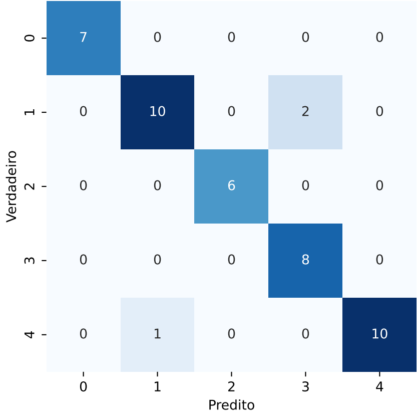
Matriz de Confusão - LDA - trabalho_6_features_bins_32-PARCIAL.csv
