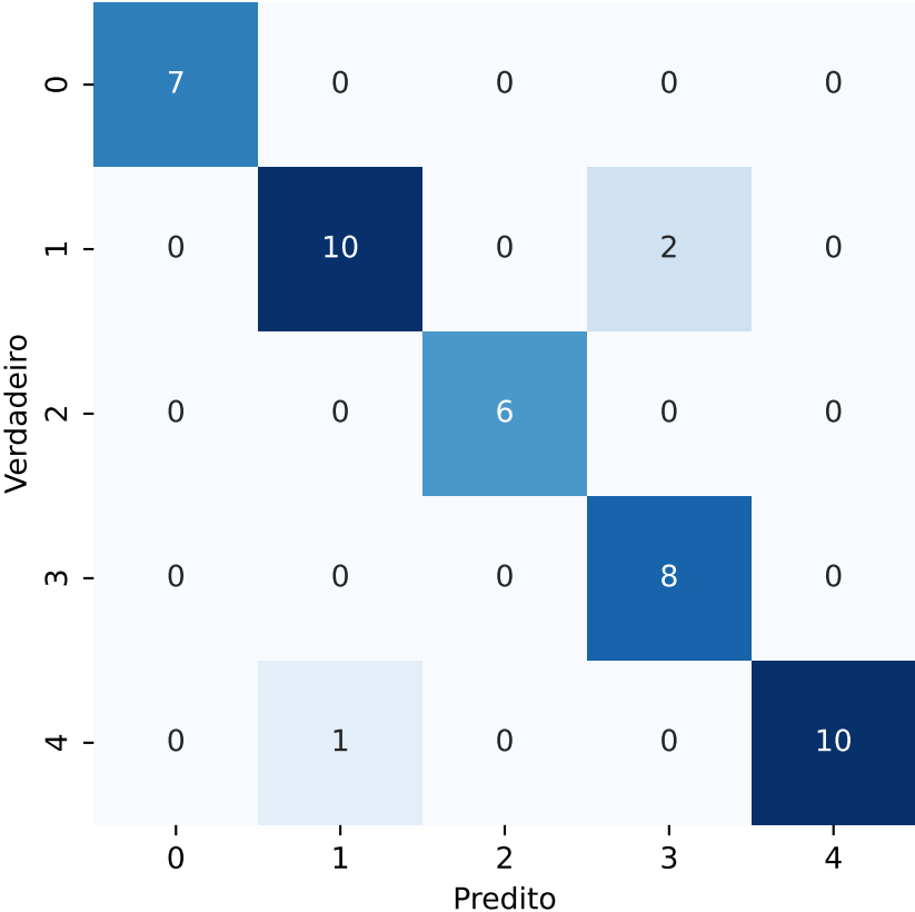
Matriz de Confusão - LDA - trabalho_6_features_bins_8-PARCIAL.csv
