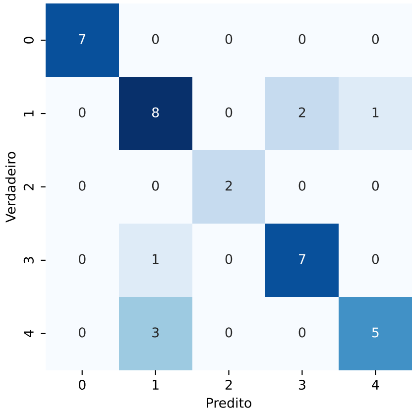
Matriz de Confusão - Naive_Bayes - trabalho_4_features_bins_32-PARCIAL.csv
