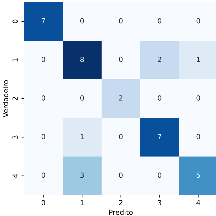
Matriz de Confusão - Naive_Bayes - trabalho_4_features_bins_8-PARCIAL.csv
