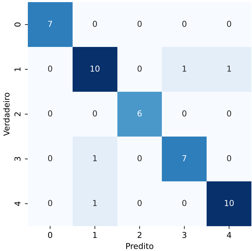
Matriz de Confusão - Naive_Bayes - trabalho_6_features_bins_32-PARCIAL.csv
