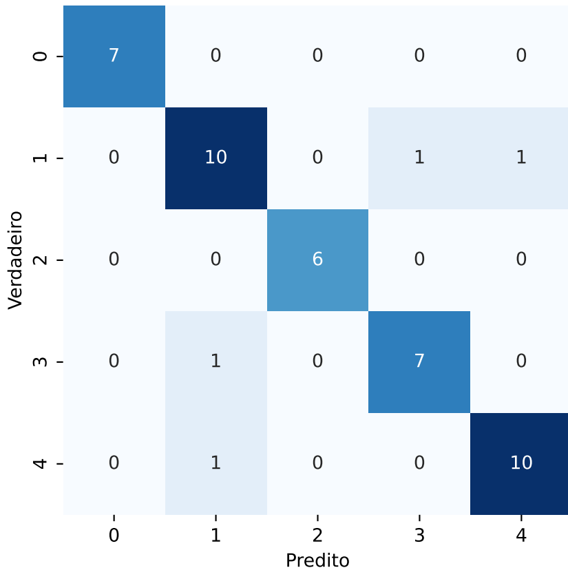
Matriz de Confusão - Naive_Bayes - trabalho_6_features_bins_8-PARCIAL.csv
