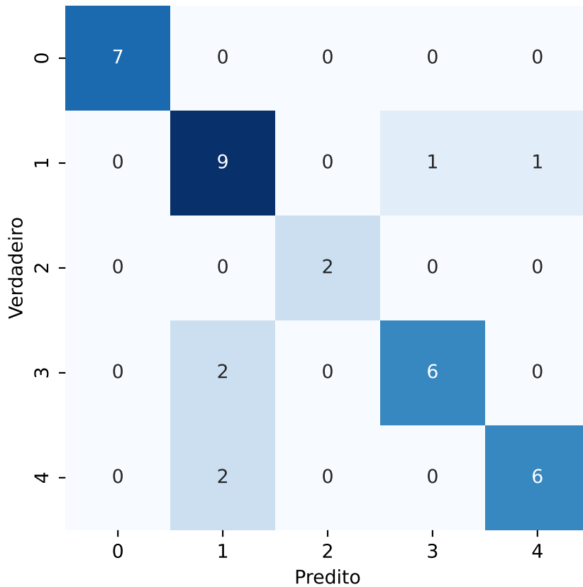
Matriz de Confusão - QDA - trabalho_4_features_bins_32-PARCIAL.csv
