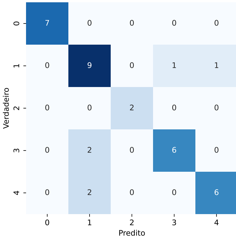
Matriz de Confusão - QDA - trabalho_4_features_bins_8-PARCIAL.csv
