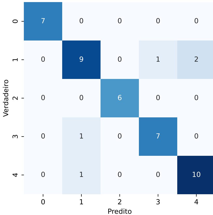
Matriz de Confusão - QDA - trabalho_6_features_bins_32-PARCIAL.csv
