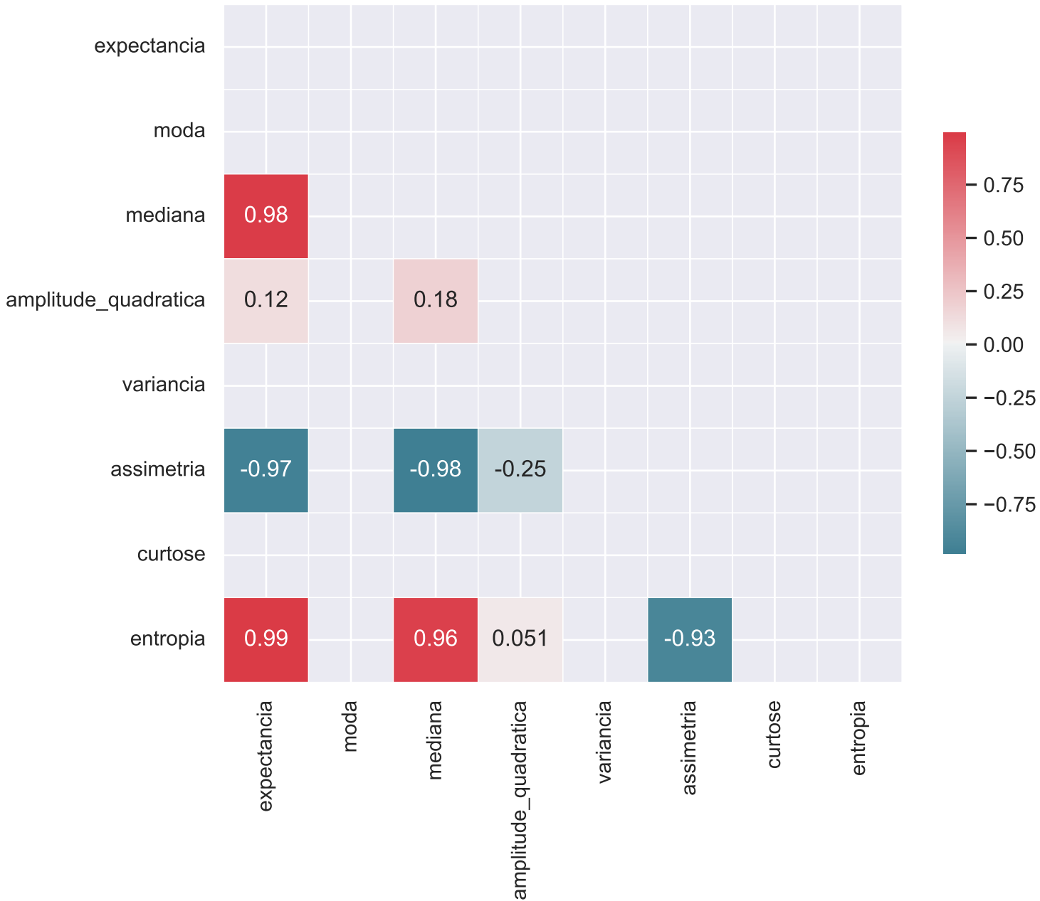
Matriz de Correlação da Classe 0 - trabalho_4_features_bins_32-PARCIAL.csv
