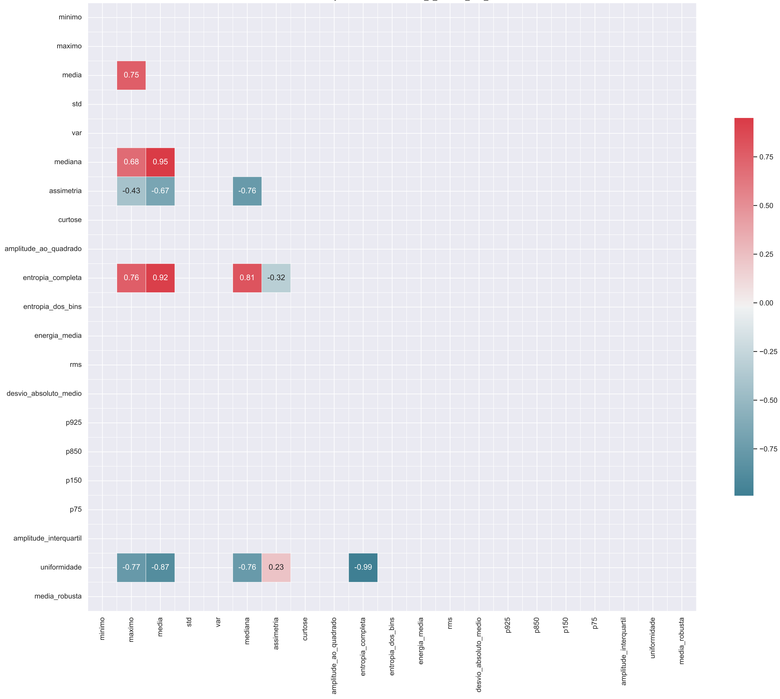
Matriz de Correlação da Classe 0 - trabalho_6_features_bins_16.csv
