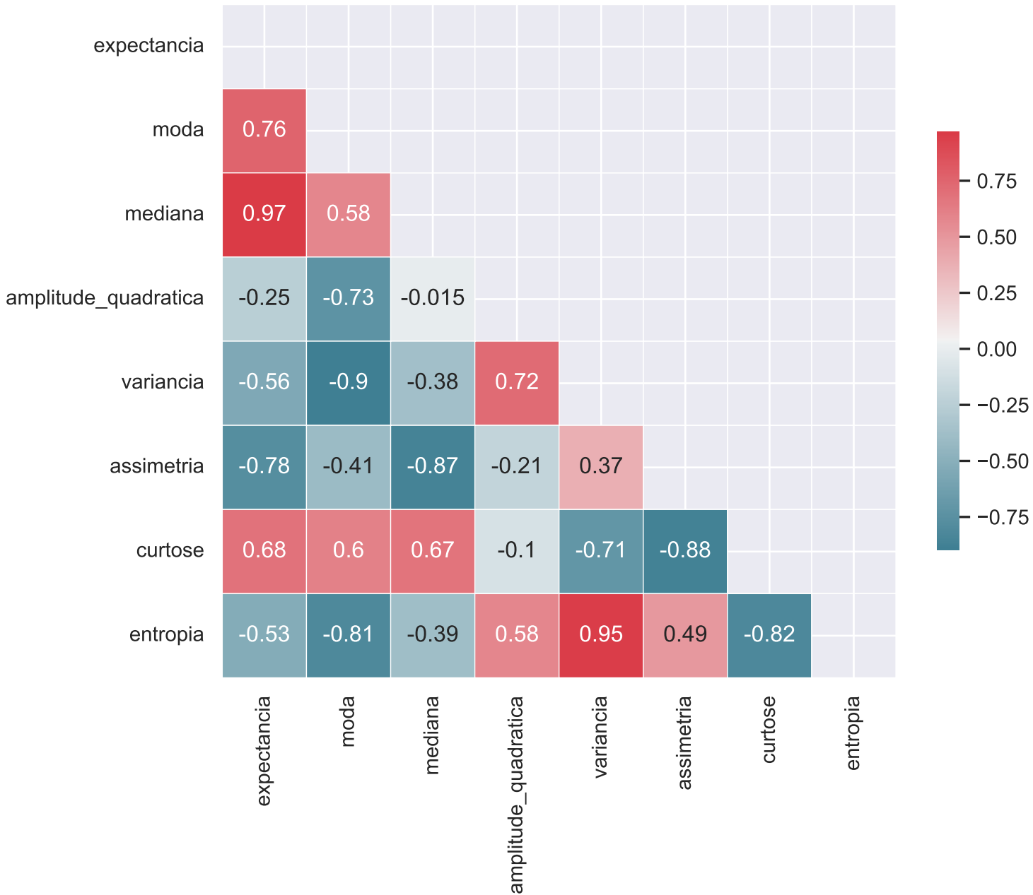
Matriz de Correlação da Classe 1 - trabalho_4_features_bins_32-PARCIAL.csv
