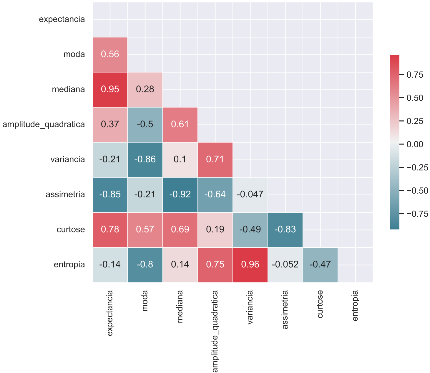
Matriz de Correlação da Classe 1 - trabalho_4_features_bins_32.csv
