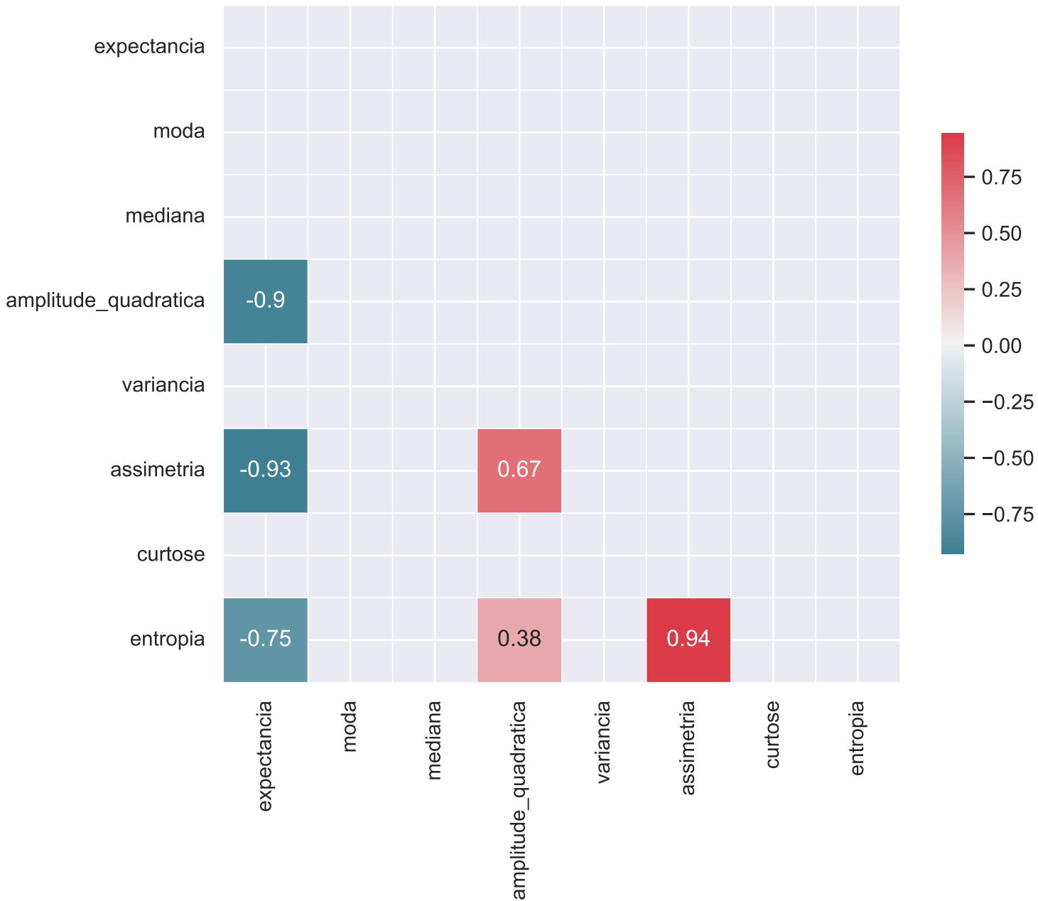
Matriz de Correlação da Classe 2 - trabalho_4_features_bins_16.csv
