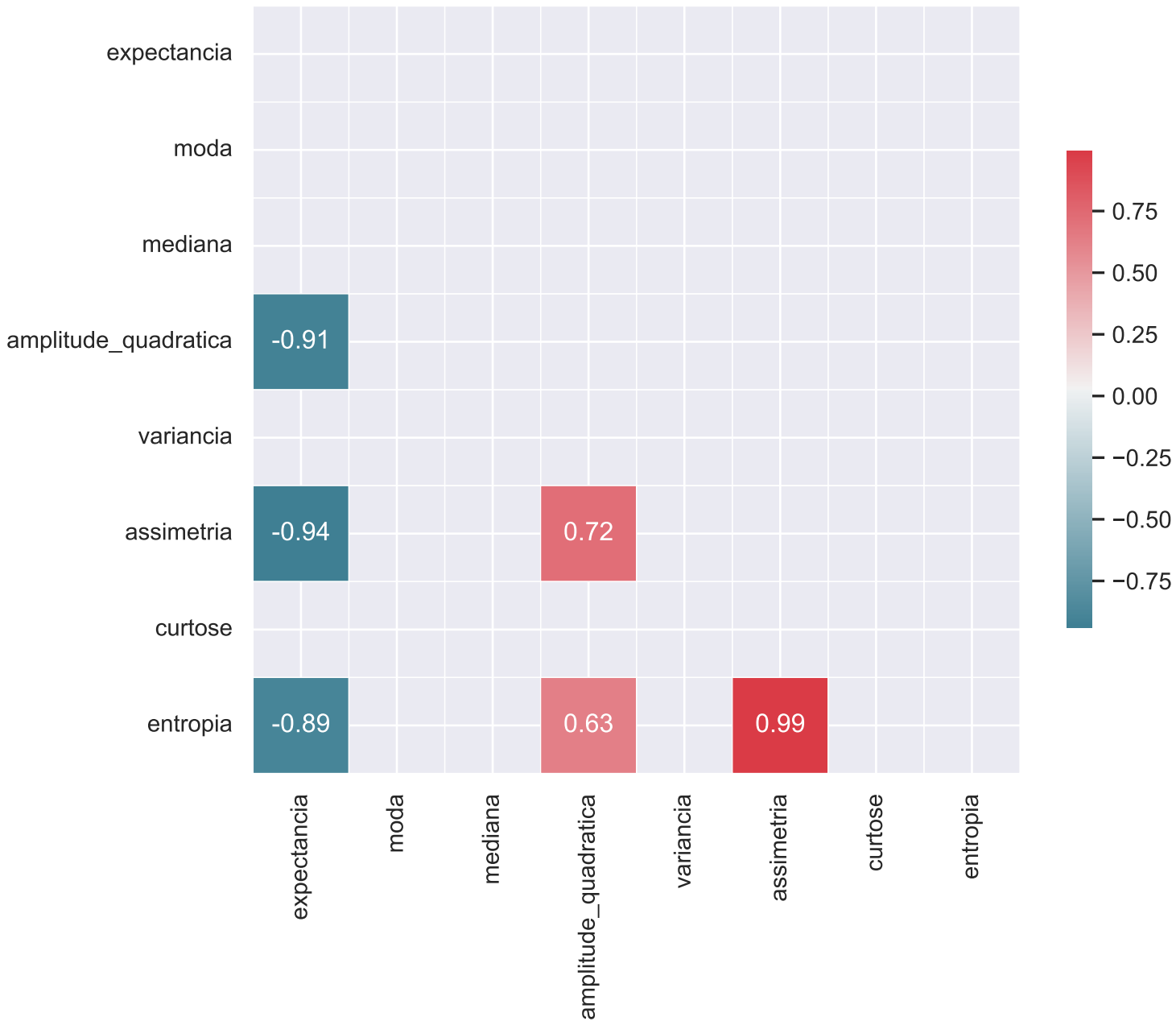
Matriz de Correlação da Classe 2 - trabalho_4_features_bins_8.csv
