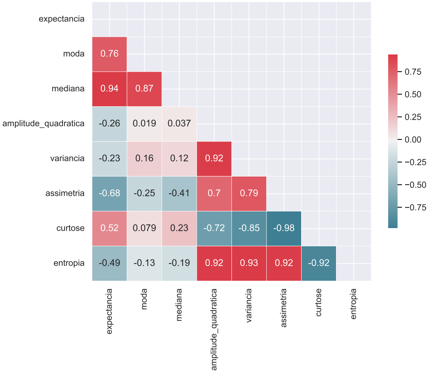
Matriz de Correlação da Classe 4 - trabalho_4_features_bins_16-PARCIAL.csv
