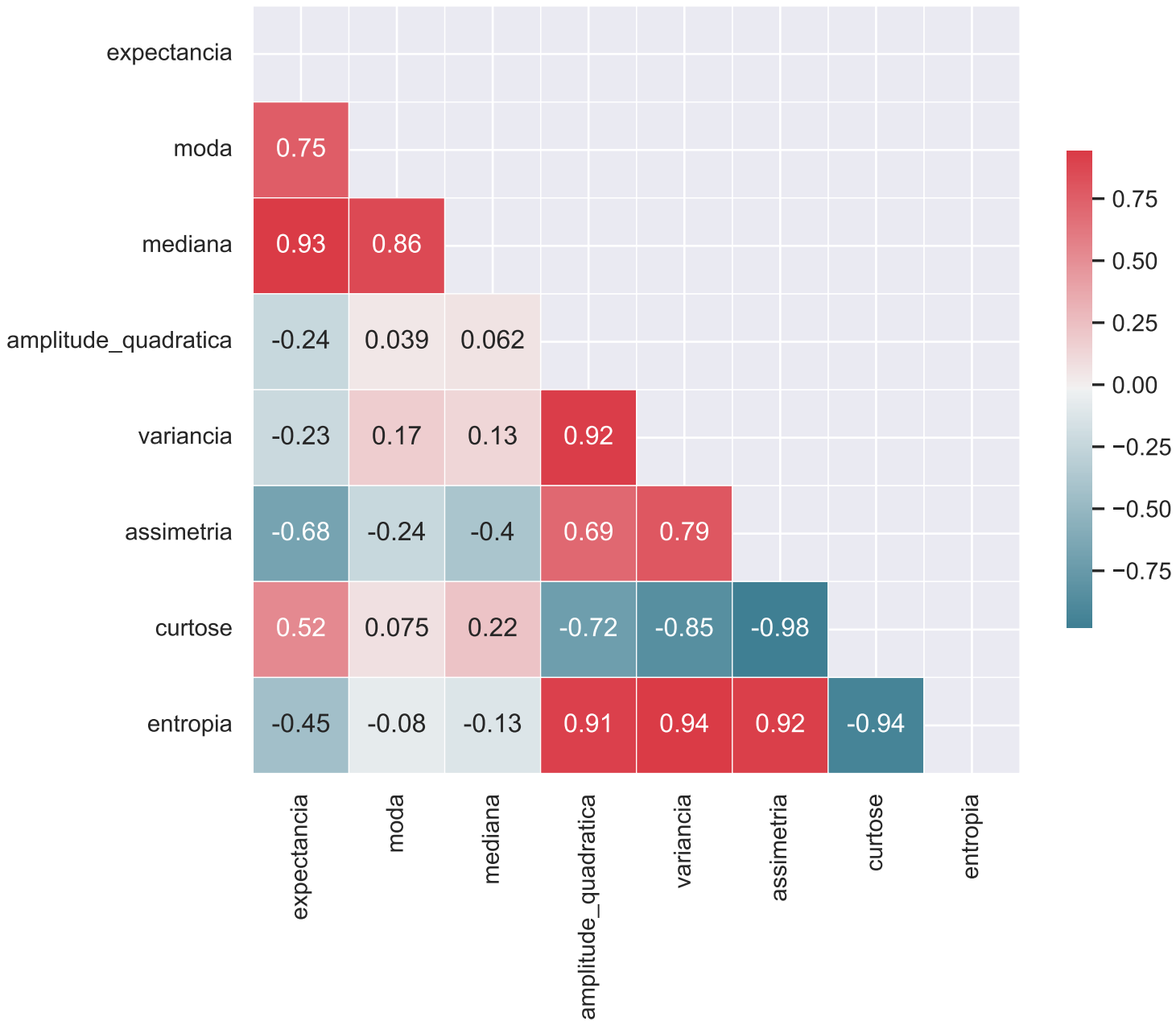
Matriz de Correlação da Classe 4 - trabalho_4_features_bins_8-PARCIAL.csv
