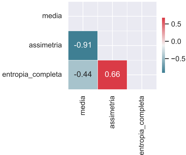
Matriz de Correlação da Classe todas - trabalho_6_features_bins_16-PARCIAL.csv
