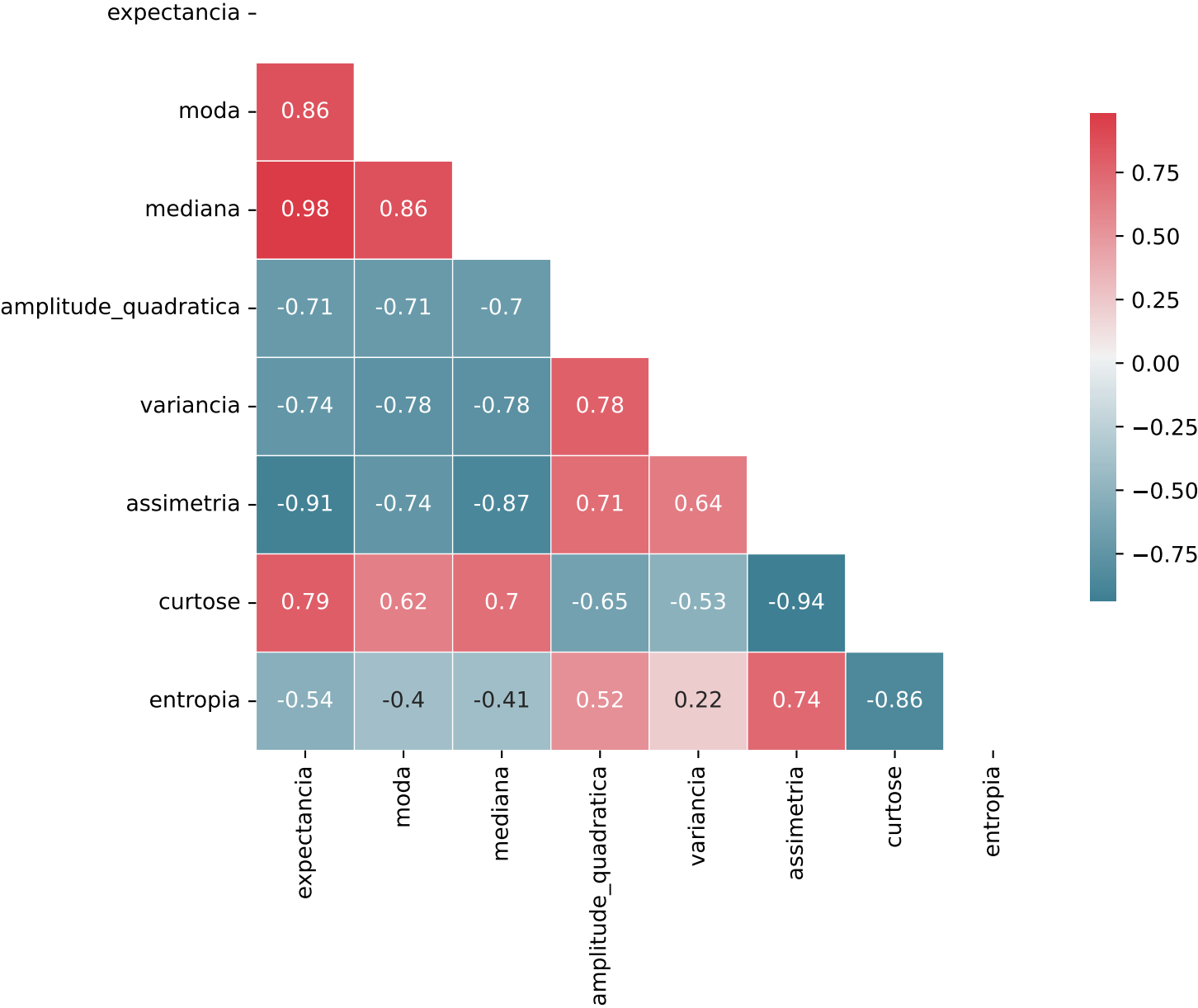
Matriz de Correlação das Features - trabalho_4_features_bins_32.csv
