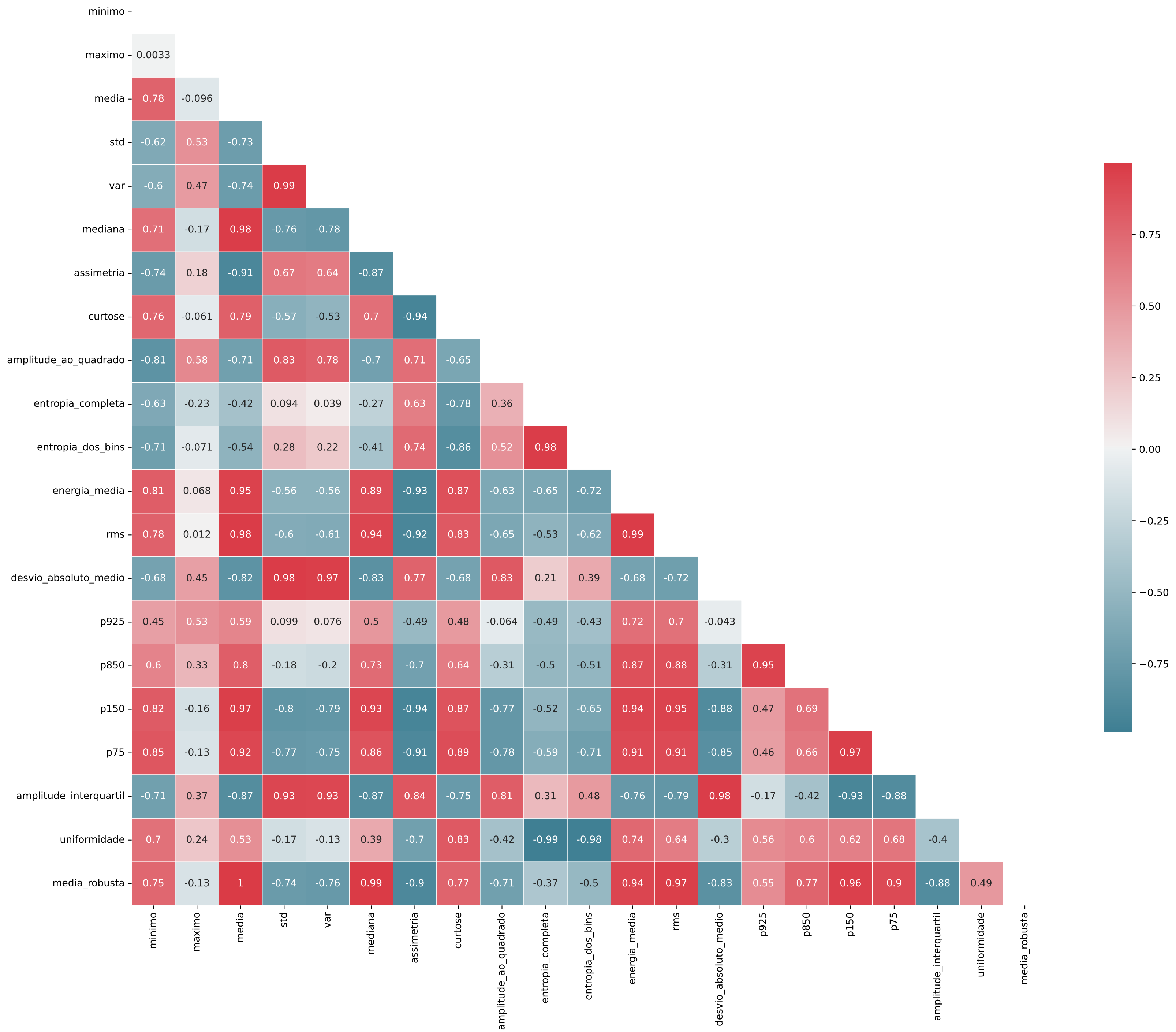
Matriz de Correlação das Features - trabalho_6_features_bins_32.csv
