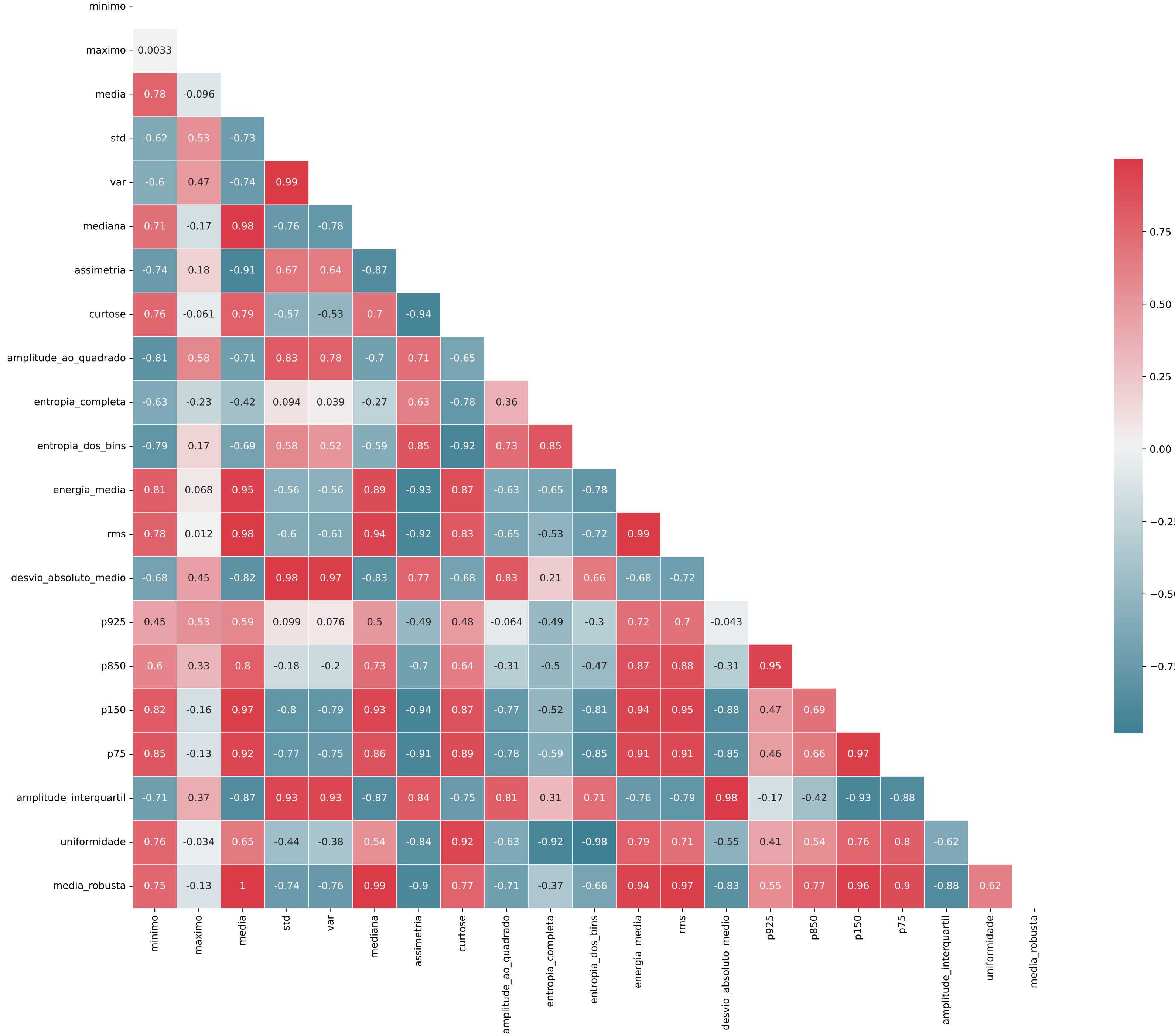
Matriz de Correlação das Features - trabalho_6_features_bins_8.csv
