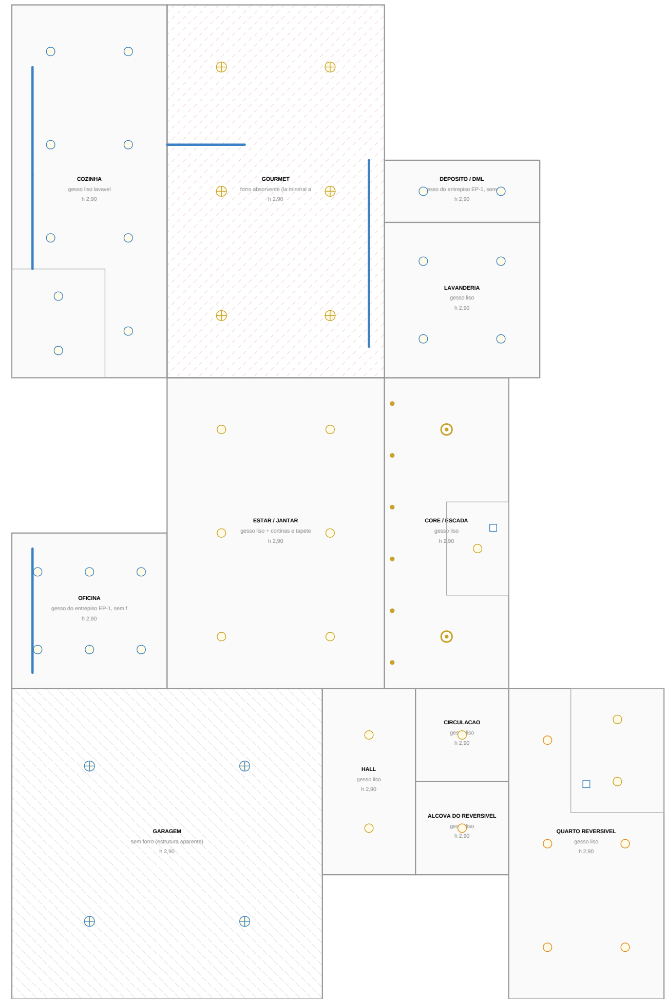
1 FORRO REFLETIDO — TERREO ESCALA 1:75
